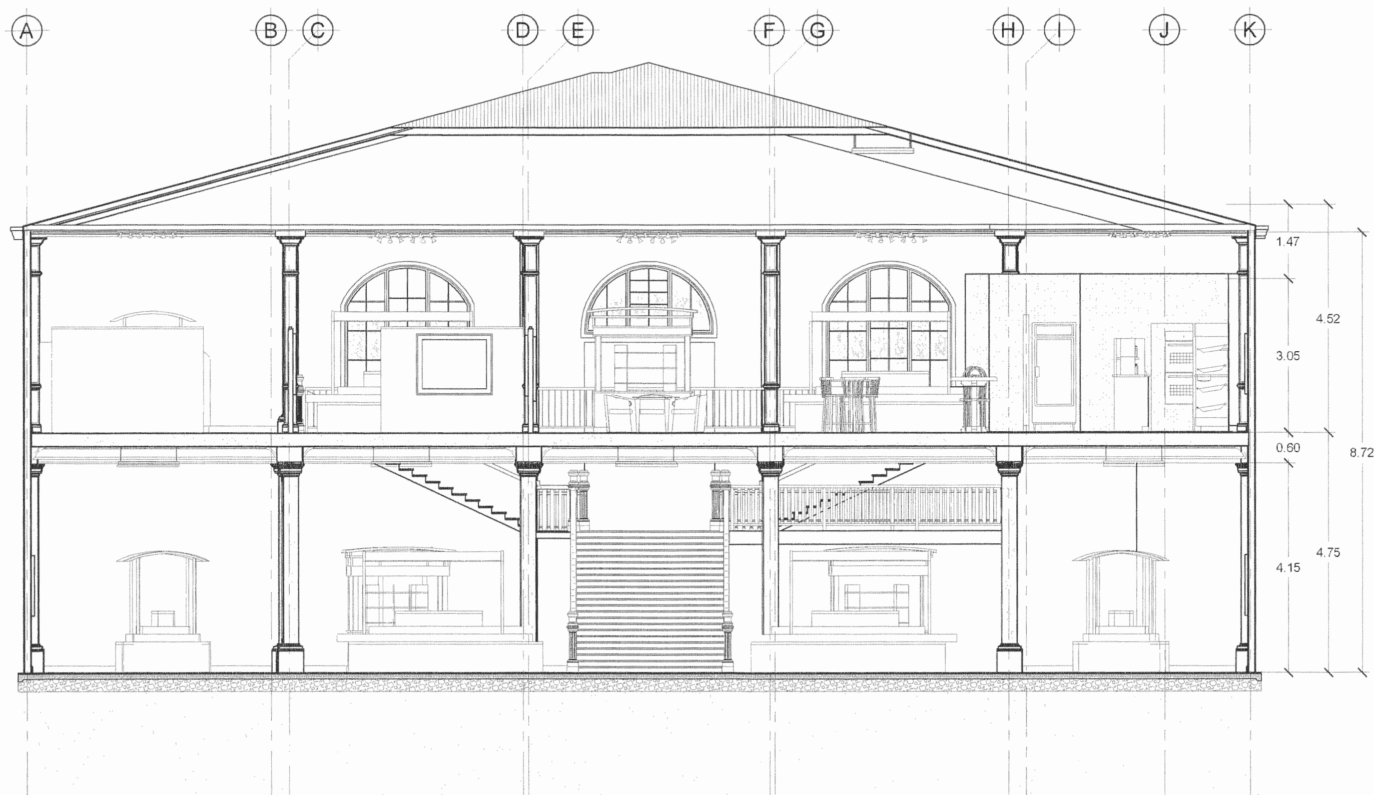
SECCION TRANSVERSAL ESCALA 1:75
