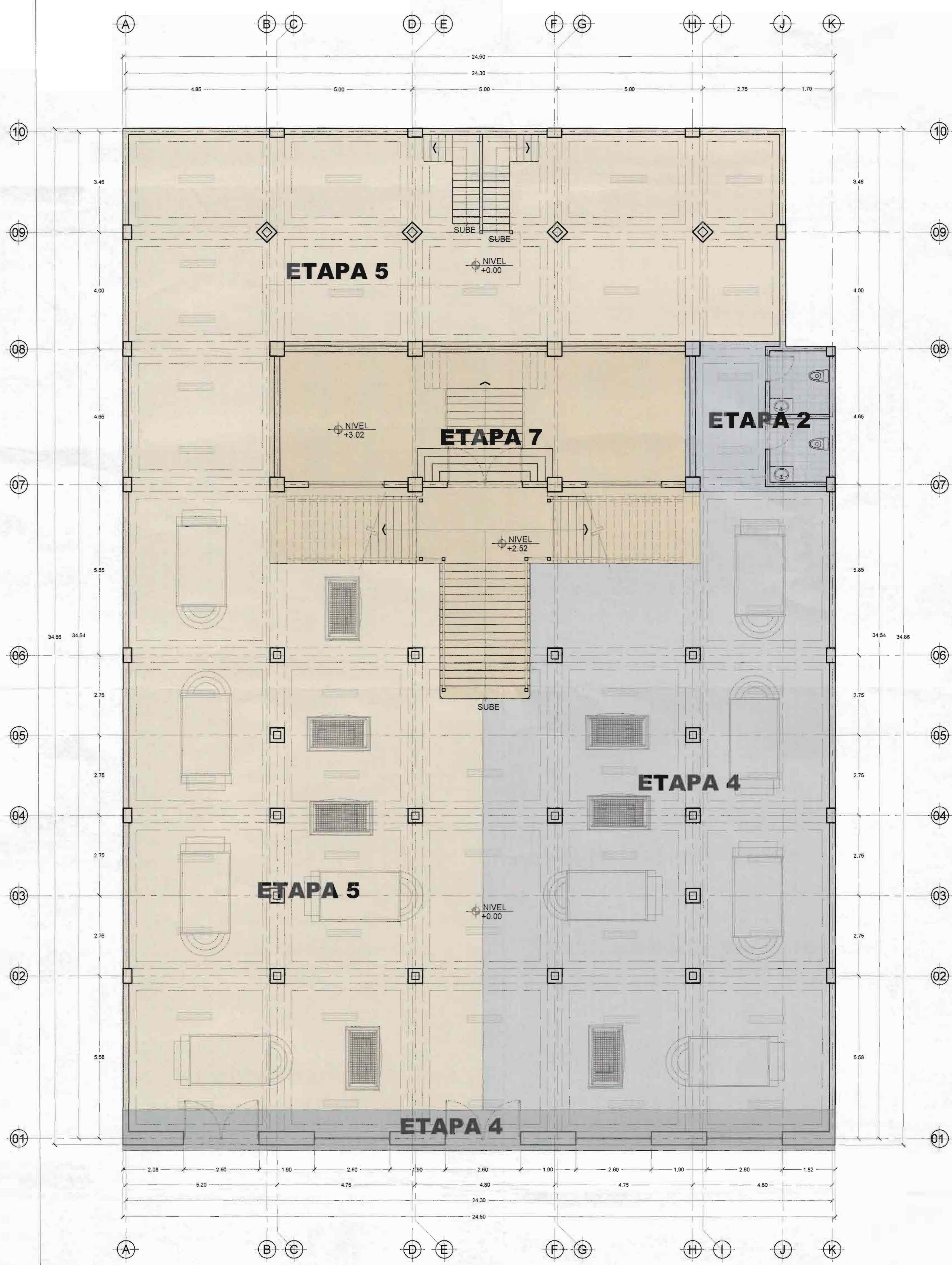
INDICACION DE ETAPAS PARA EL PROCESO DE RESTAURACION NIVEL 1 +0.00mts ESCALA 1:75
