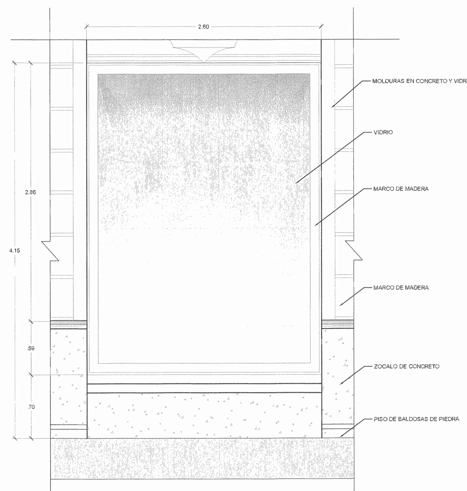
DETALLE DE VENTANA TIPICA ESCALA 1:25
