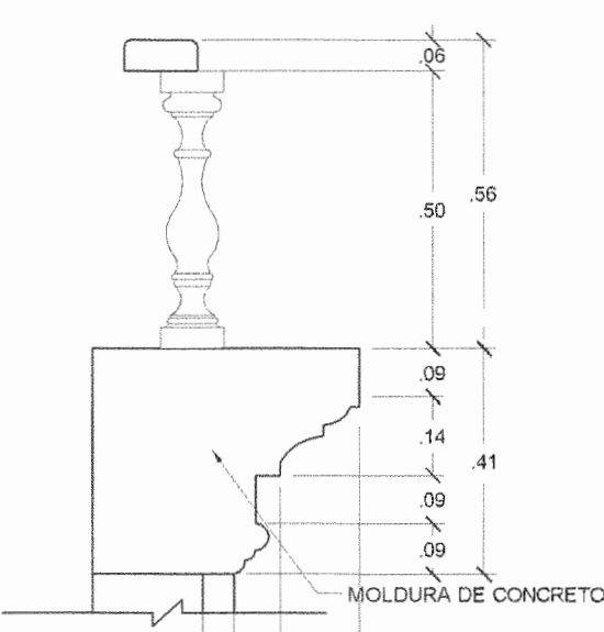
SECCION
