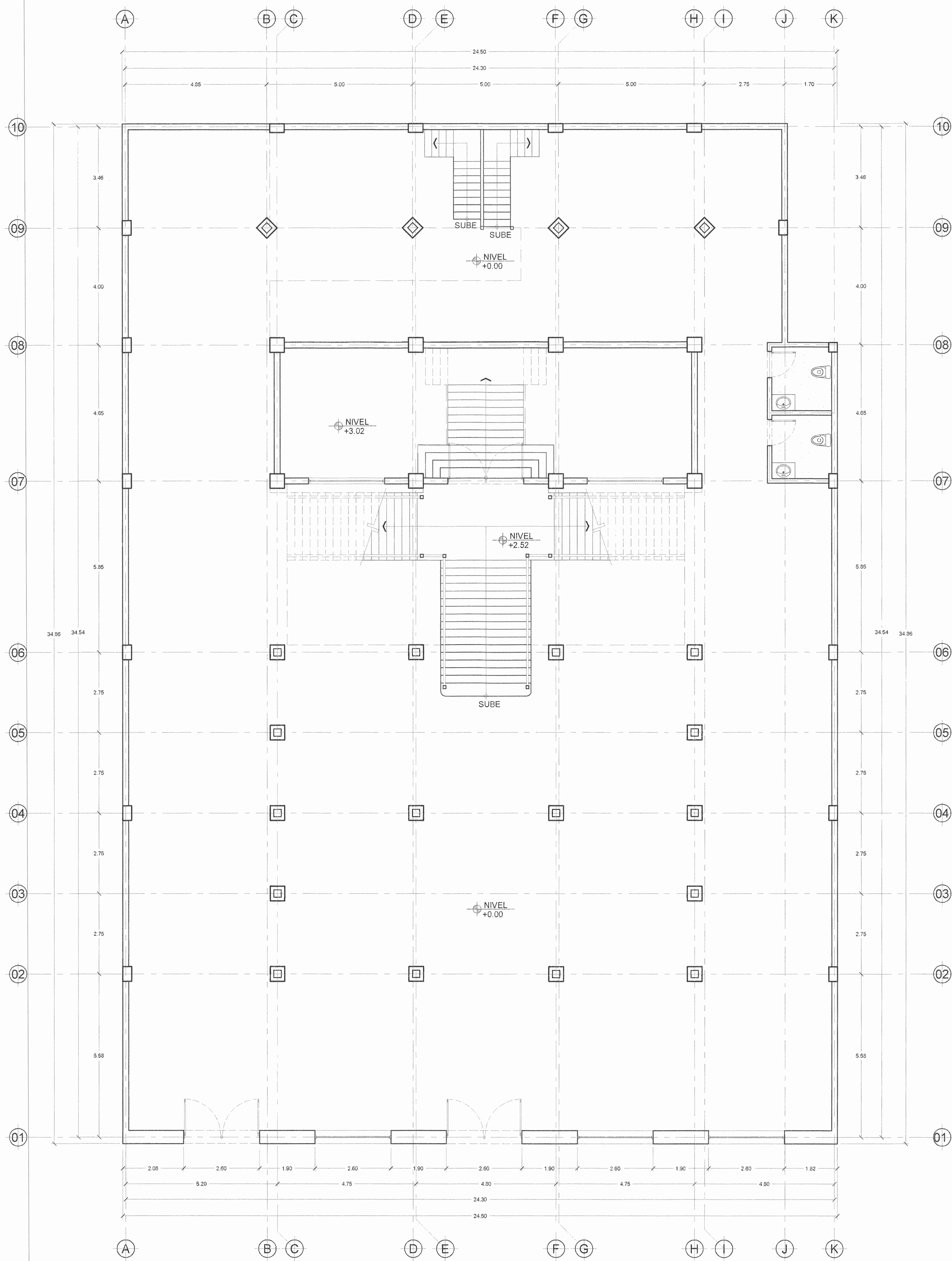
PLANTA DE DISTRIBUCION ARQUITECTONICA NIVEL 1 +0.00mts EDIFICIO EXISTENTE ESCALA 1:75
