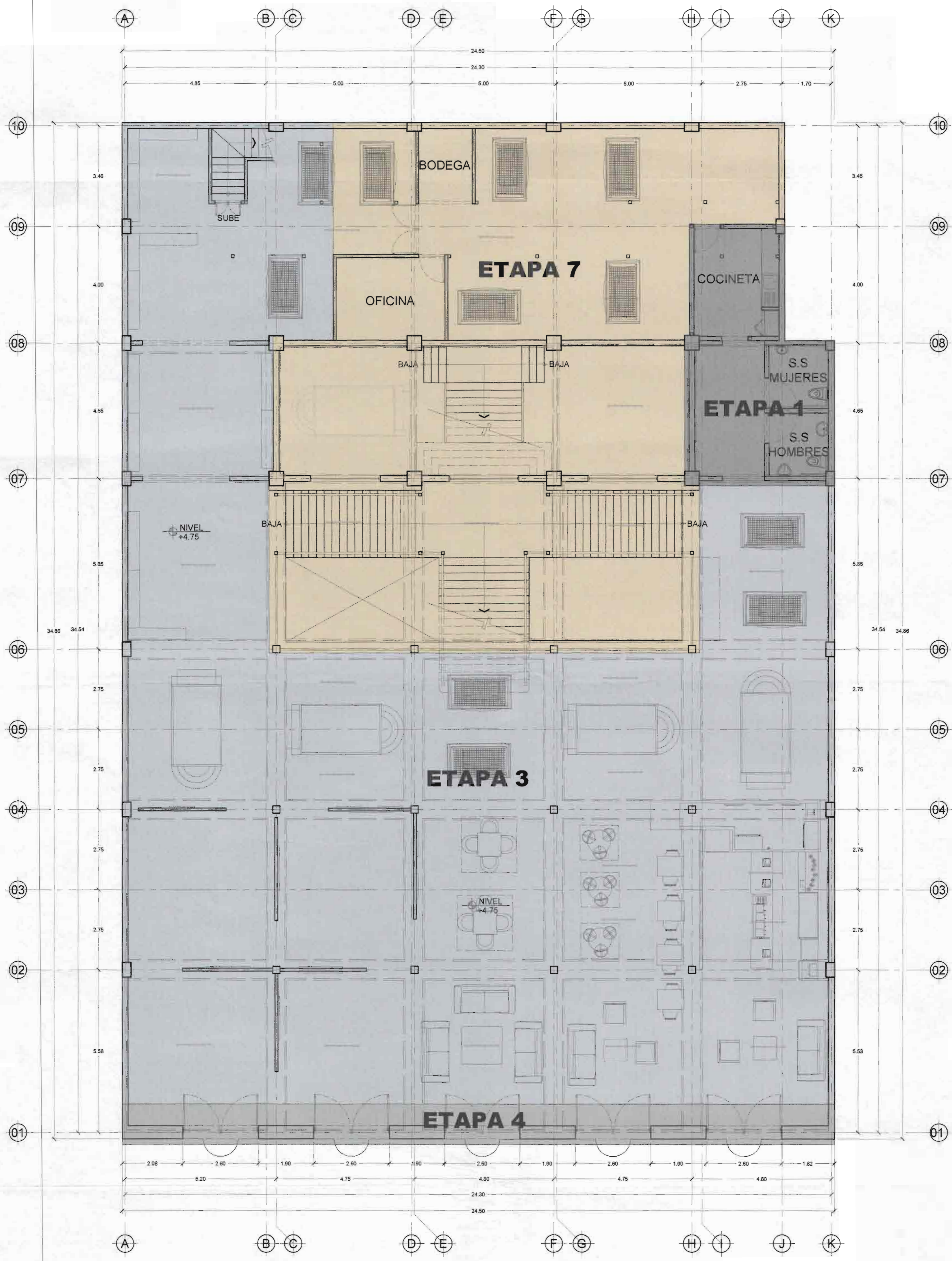
INDICACION DE ETAPAS PARA EL PROCESO DE RESTAURACION NIVEL 2 +4.75mts ESCALA 1:75
