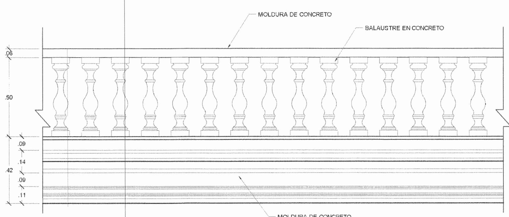
ELEVACION
