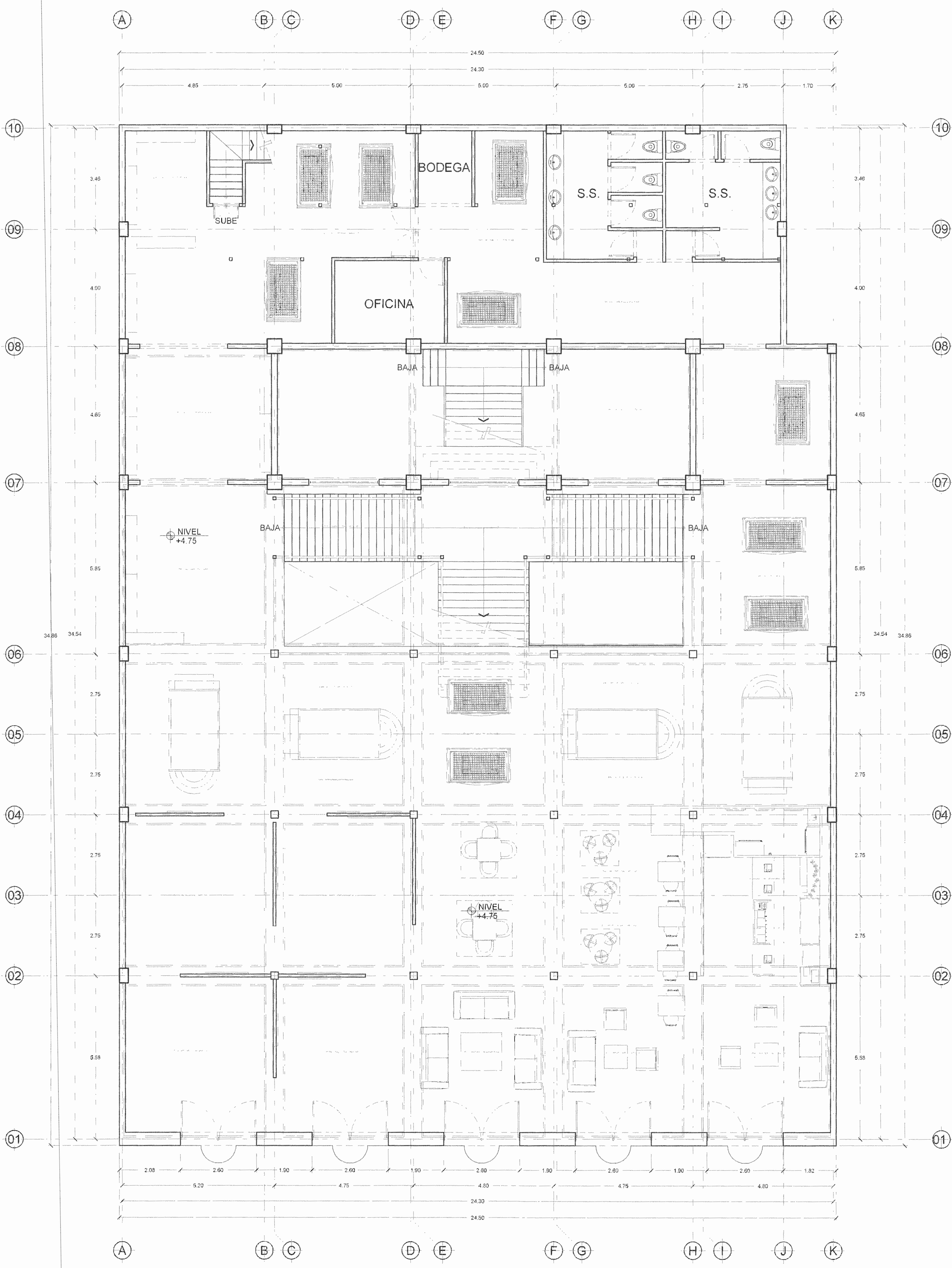
PLANTA DE DISTRIBUCION ARQUITECTONICA NIVEL 2 +4.75mts PROPUESTA ARQUITECTONICA ESCALA 1:75
