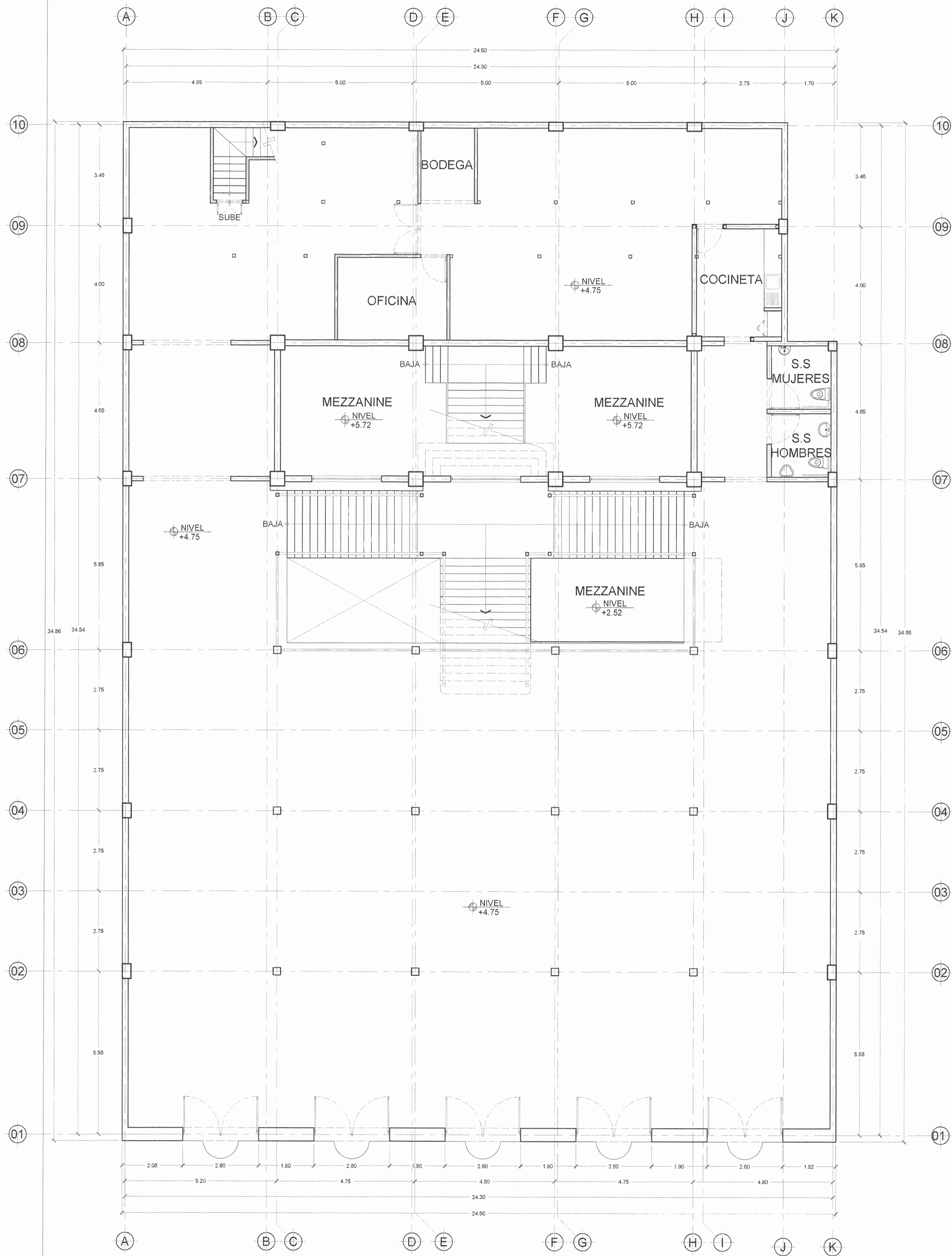
PLANTA DE DISTRIBUCION ARQUITECTONICA NIVEL 2 +4.75mts EDIFICIO EXISTENTE ESCALA 1:75
