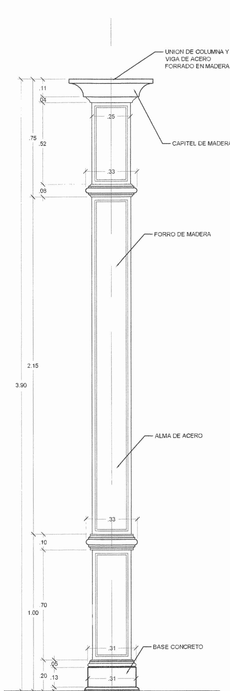
ELEVACION
