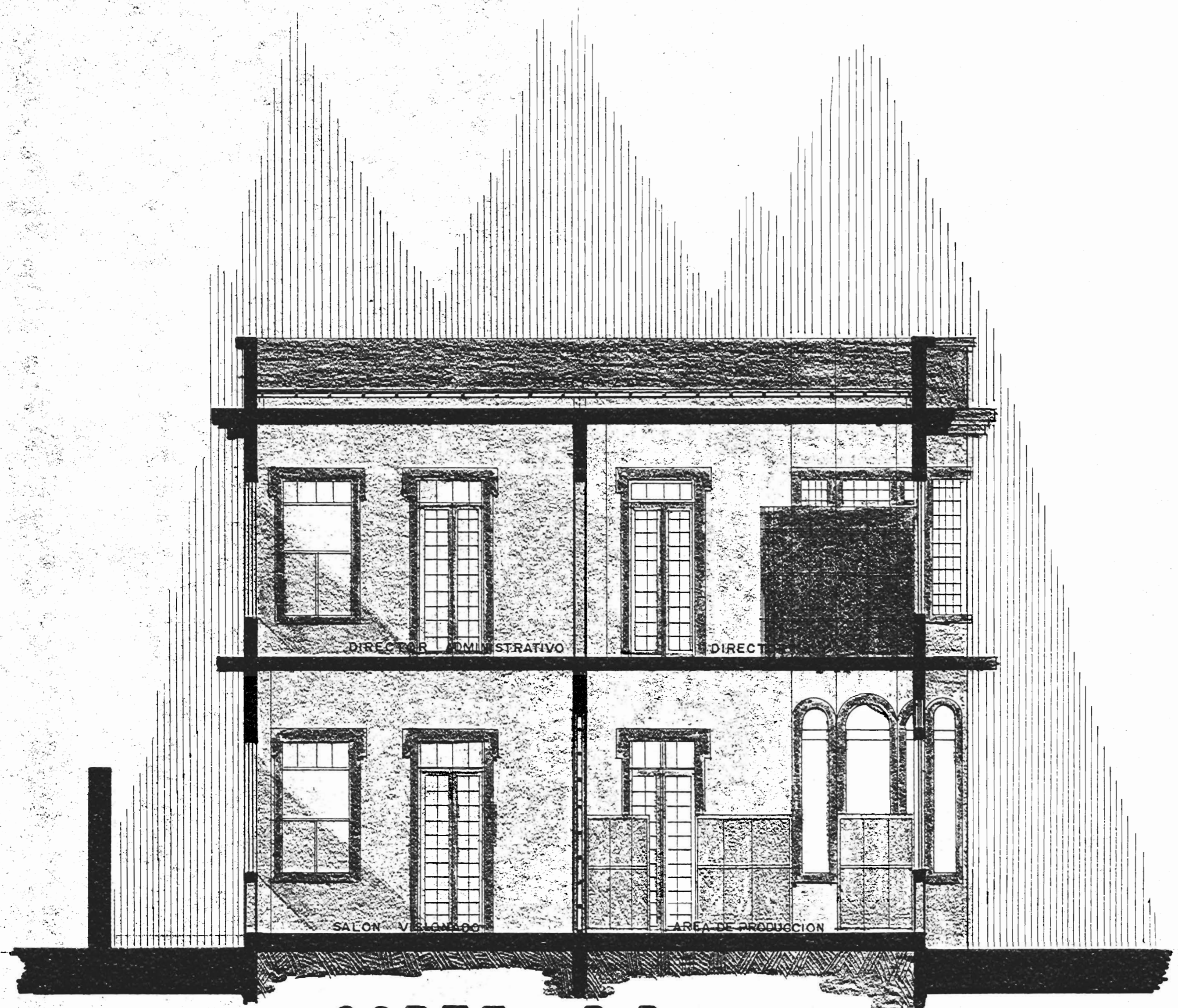
CORTE B-B ESCALA 1:50
