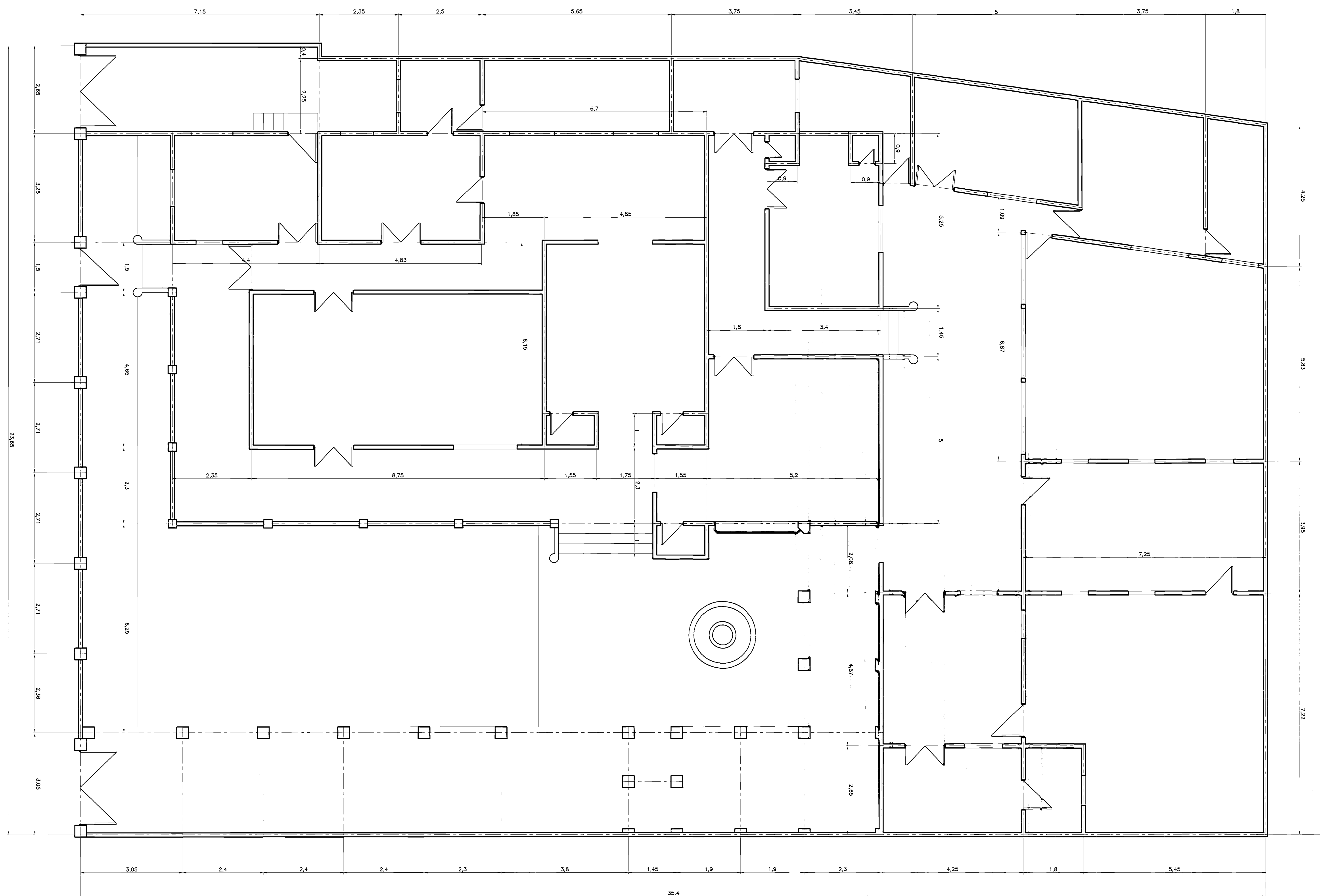
PLANTA DE DISTRIBUCION ARQUITECTONICA PRIMER NIVEL
