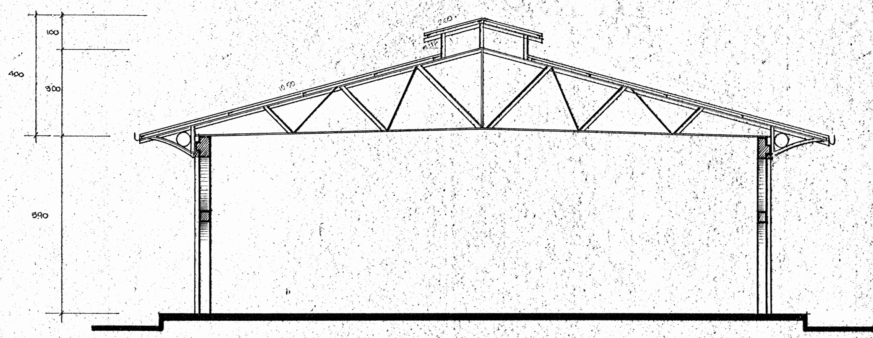
CORTE TRANSVERSAL
