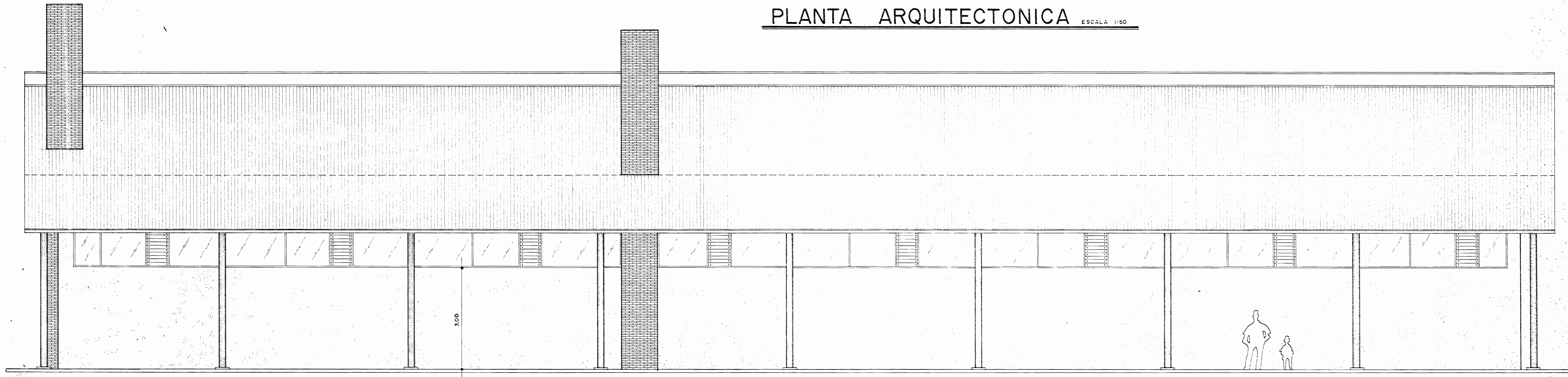
ALZADO OESTE ESCALA 1:50
