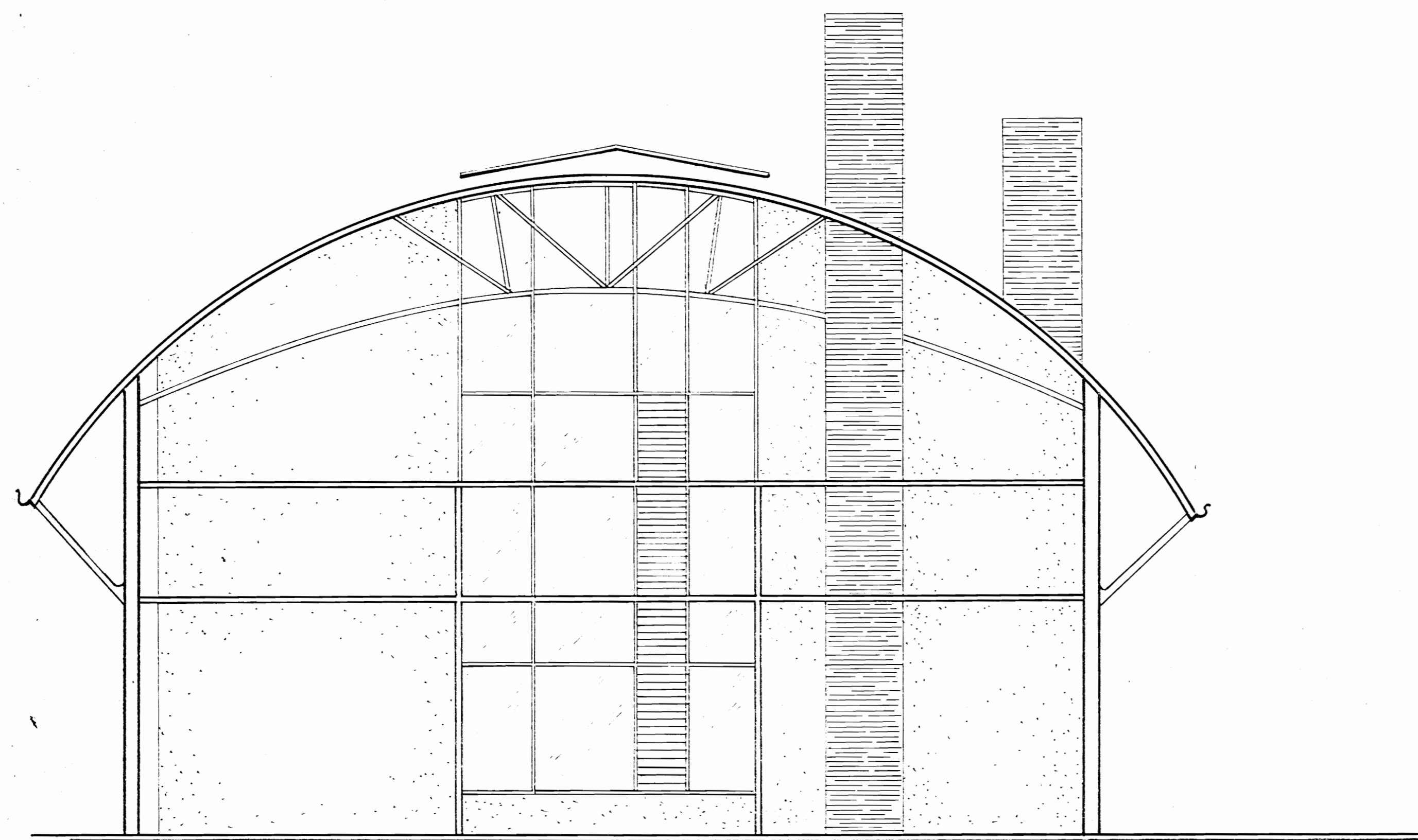
FACHADA NORTE ESCALA: 1:50
