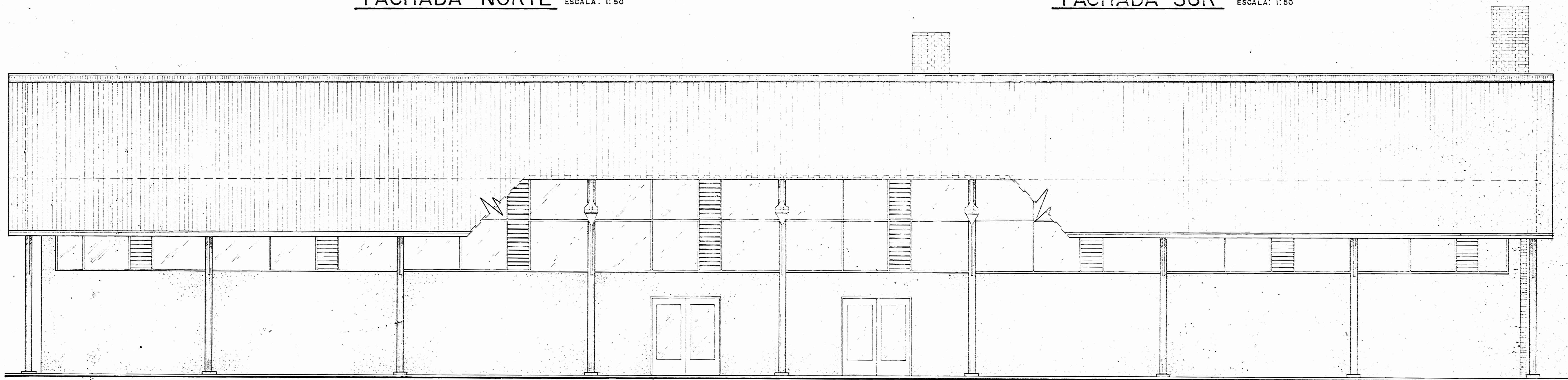
FACHADA NORTE ESCALA: 1:50
