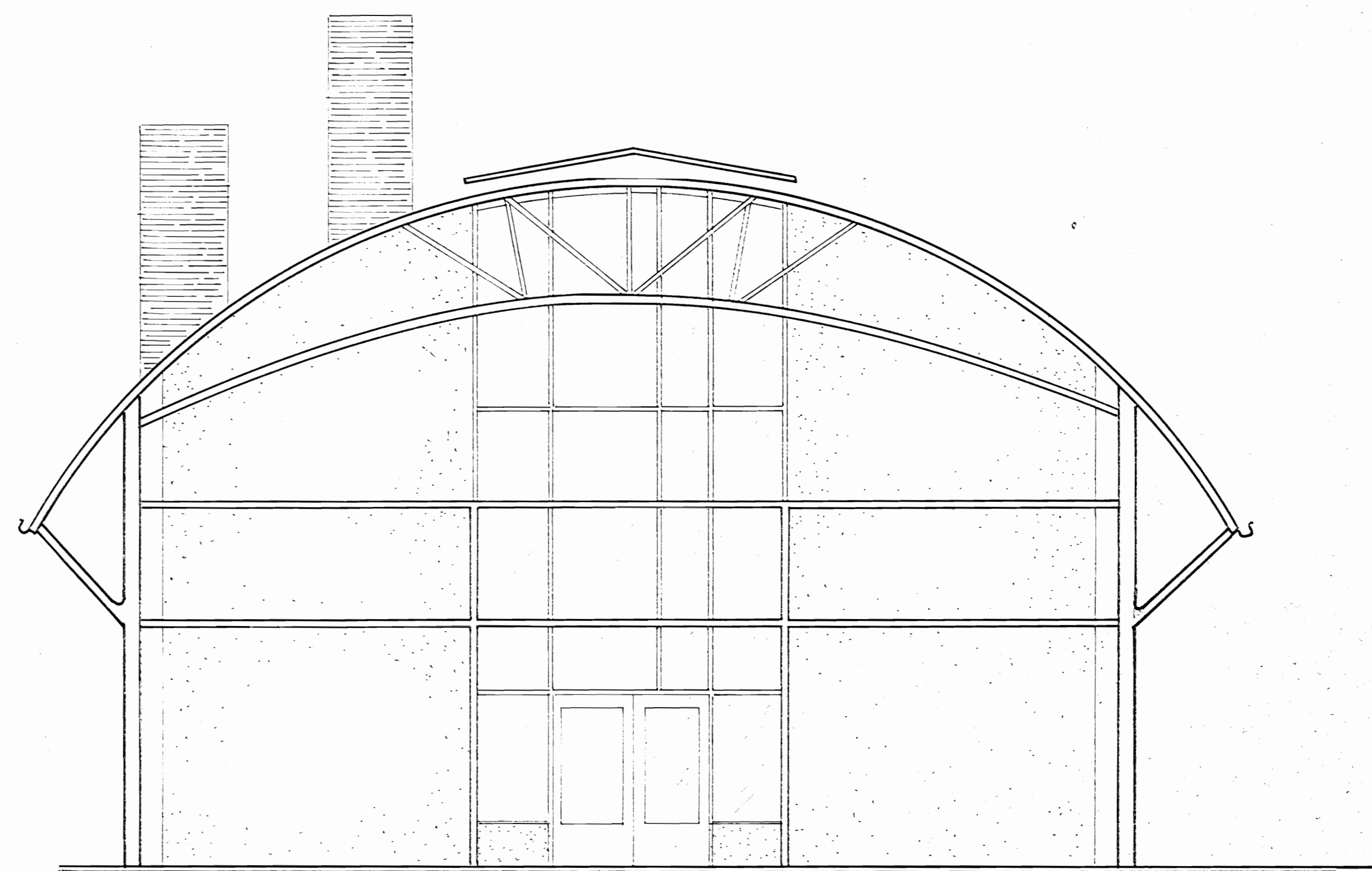
FACHADA SUR ESCALA: 1:50
