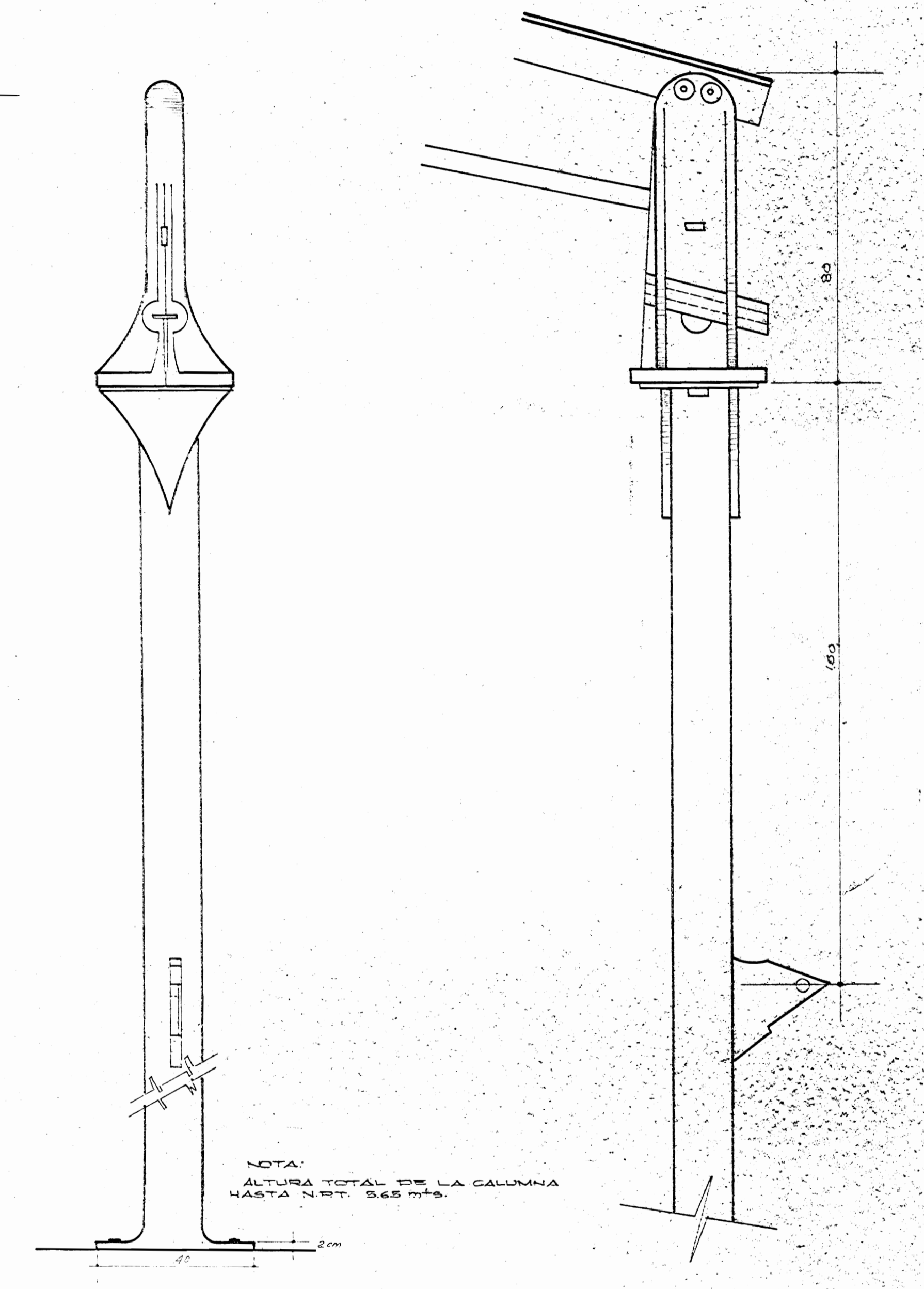
DETALLE DE COLUMNA (FRENTE Y PERFIL) ESC 1:10
