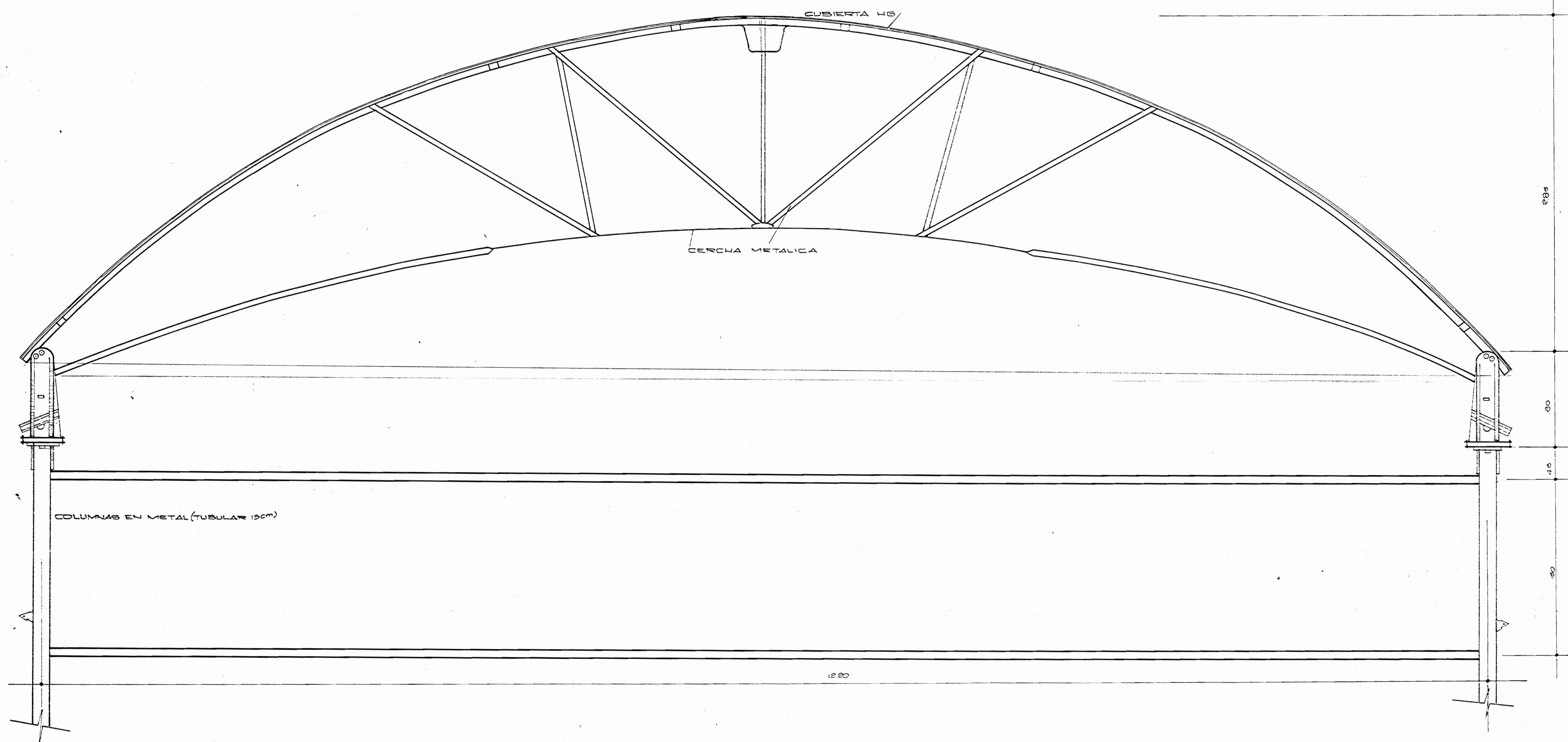
DETALLE DE CERCHA Y COLUMNA ESCALA 1:20
