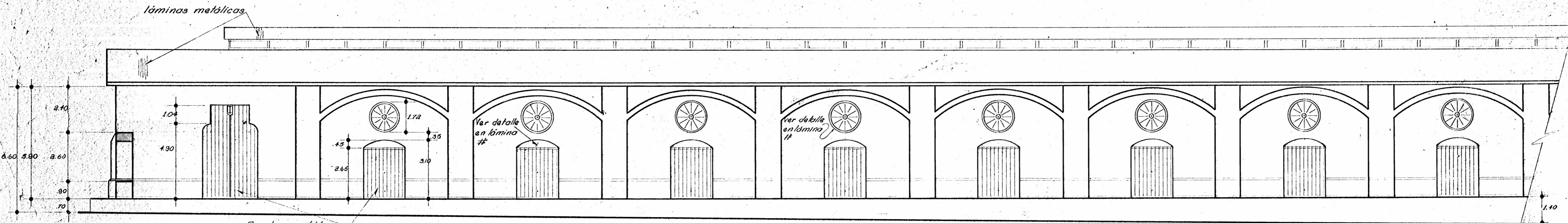
FACHADA OESTE escala 1:100
