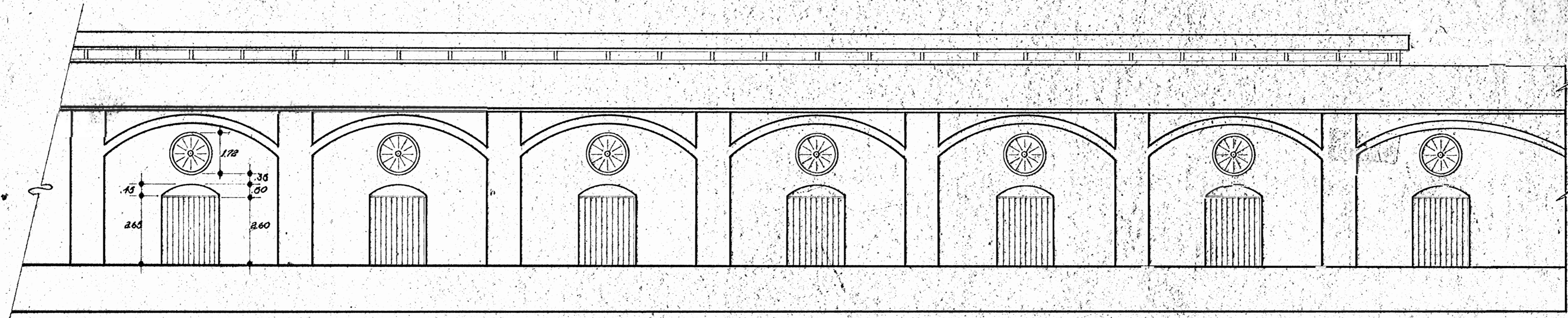
FACHADA OESTE escala 1:100
